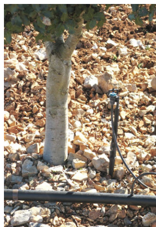
Micro-aspiration appliquée en trufficulture
