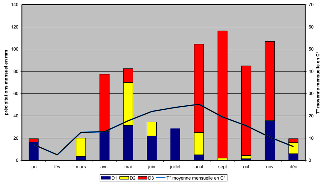
Ombrothermique Montségur/Lauzon 2012
